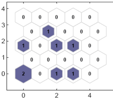
Рис. 8. Діаграма влучень прикладів у нейрони гексагональної конфігурації
