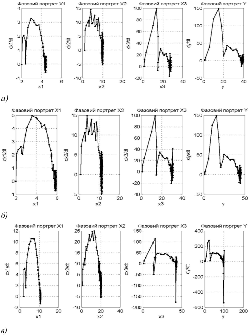
Рис. 6. Фазові портрети біфуркаційних діаграм моделі: сценарій ЖЦП а), б), в) розквіт
