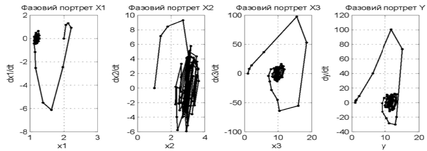
Рис. 5. Фазові портрети біфуркаційних діаграм моделі: сценарій ЖЦП а), б) зрілість
