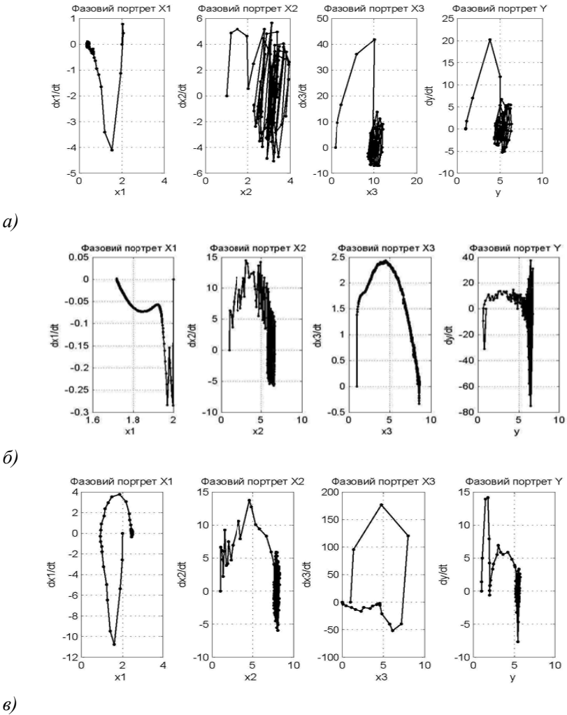
Рис. 4. Фазові портрети біфуркаційних діаграм моделі: сценарії ЖЦП а) летальна, б) народження, в) розвиток
