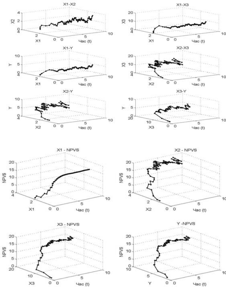
Рис. 3. Параметричні діаграми моделі (сценарій ЖЦП «летальна»)
