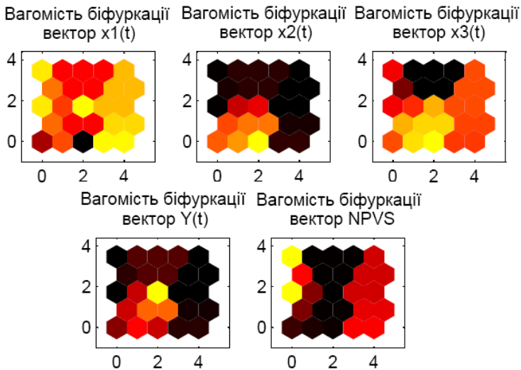
Рис. 7. Компонентні фігури вагових позицій параметрів стану біфуркації ЖЦП підприємств
