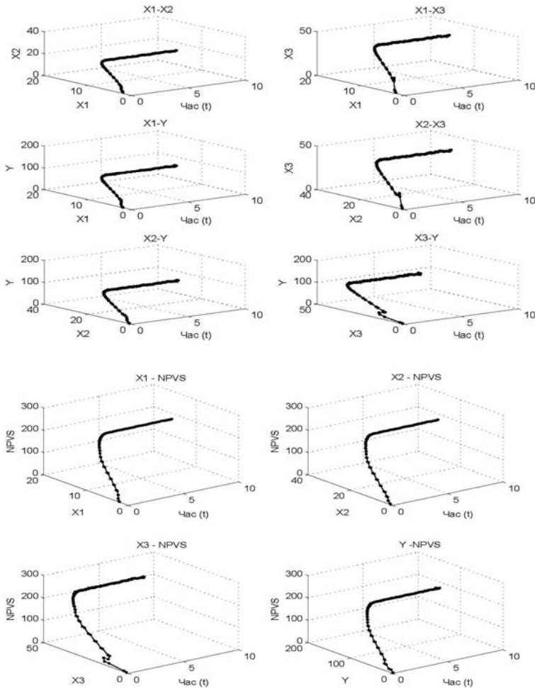
Рис. 2. Параметричні діаграми моделі (сценарій ЖЦП «розквіт»)
