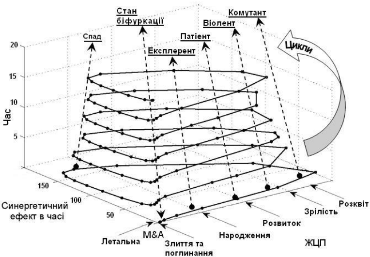
Рис. 1. Тривимірний фазовий портрет життєвого циклу розвитку підприємства
