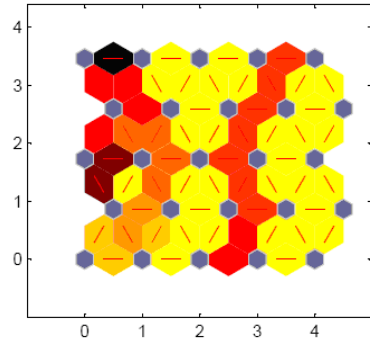
Рис. 9. Уніфікована матриця відстаней
